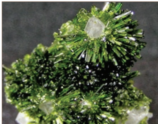
Figura 37 - Epidoto
